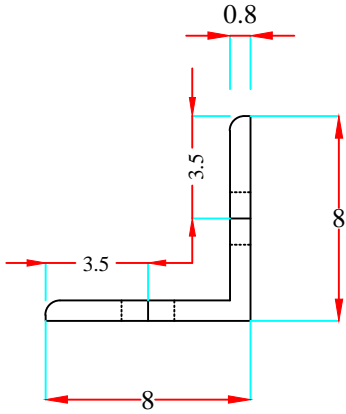
نمای کنسول از بغل
